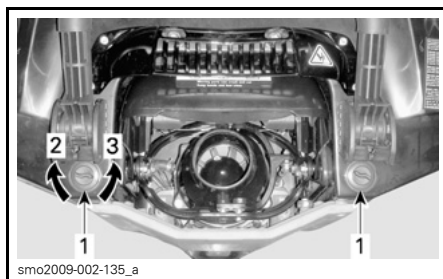
TYPEBILDE – PLASSERING AV DRENERINGSPLUGGER FOR BUNNVANN 1. Dreneringsplugger for bunnvann 2. Trekk til 3. Åpne
