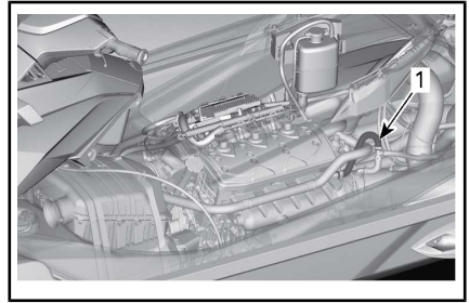
1. Tubo flessibile
