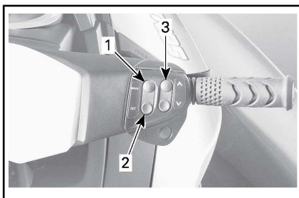
CONFIGURAZIONE TIPICA - PULSANTI DI CONTROLLO DELL'INDICATORE
