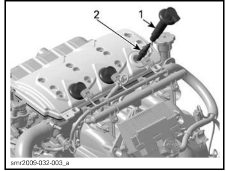
1. Bobine d'allumage 2. Bougie
