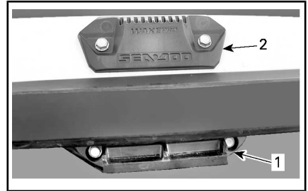
SOPORTE DE SUJECIÓN PARA EL PORTATABLAS DE WAKEBOARD
