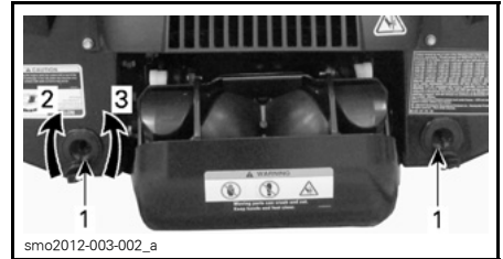
TYPEBILDE – PLASSERING AV DRENERINGSPLUGGER FOR BUNNVANN
