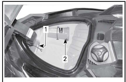
OPBERGVAK VOORAAN
