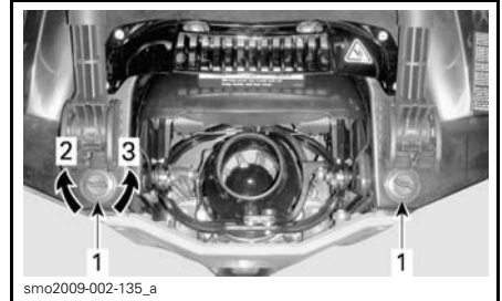
TYPIQUE - EMPLACEMENTS DES BOUCHONS DE VIDANGE DE CALE
