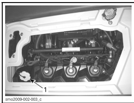
TÍPICO 1. Ubicación del tapón de llenado de aceite
