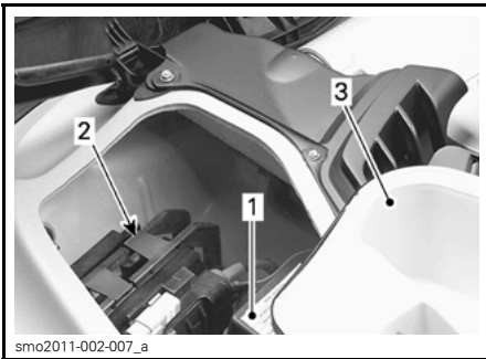
TÍPICO 1. Caja de fusibles 2. Soporte de batería 3. Contenedor de almacenamiento
