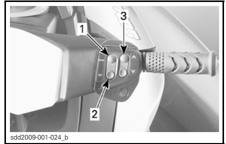
TÍPICO - BOTONES DE CONTROL DE INDICADORES
