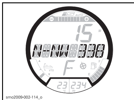
AFFICHAGE MULTIFONCTIONNEL - INFORMATION PROVENANT DE LA BOUSSOLE
