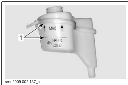
smo2009-002-137_a TYPIQUE - RÉSERVOIR D'EXPANSION DU SYSTÈME DE REFRIGÉREMENT 1. Niveau entre les marques alors que le moteur est froid
