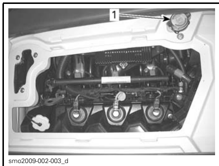
smo2009-002-003_d TYPIQUE - MODÈLE RXT iS ILLUSTRÉ 1. Bouchon de réservoir d'expansion
