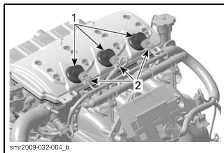
smr2009-032-004_b 1. Bobine d'allumage 2. Connecteur de bobine d'allumage
