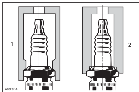
1. Douille approuvée 2. Douille inadéquate
