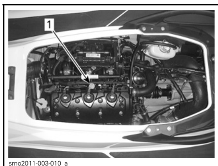
代表的な例 - RXT iS の場合 1. オイルレベルゲージの位置
