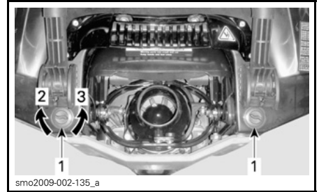
TÍPICO - LOCALIZAÇÕES DOS BUJÕES DE DRENAGEM DO BOJO
