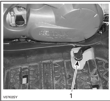
1. Rempedaal
