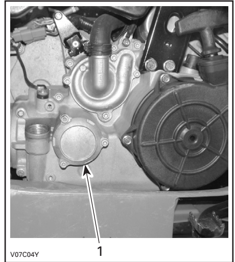
TYPISCH 1. Oliefilterdeksel
