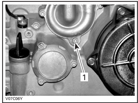
1. Koelvloeistof-aftapplug
