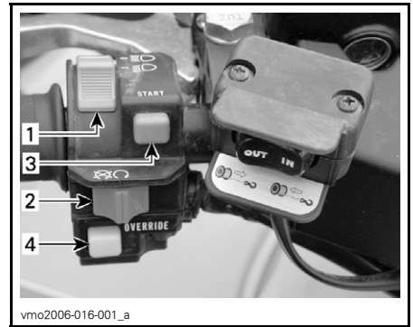
TÍPICO — INTERRUPTOR MULTIFUNCIÓN
