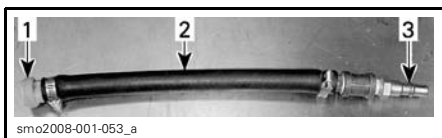
TYPIQUE 1. Adaptateur de raccord de rinçage (N/P 295 500 473) 2. Boyau 12.7 mm (1/2 po) 3. Adaptateur mâle de boyau d'air
