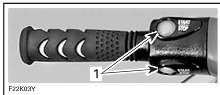
1. Motorstart/stopknoppen
