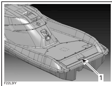
1. Rompidentificatienummer
