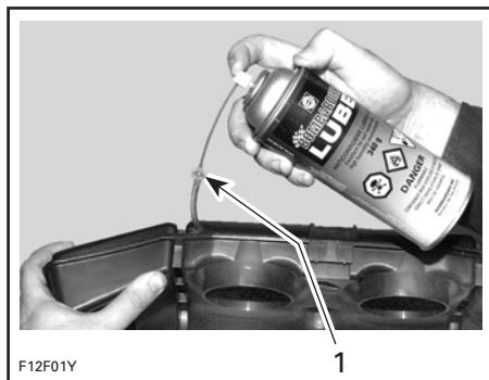
1. Tirer partiellement le tube hors du silencieux d'admission d'air pour injecter le lubrifiant XP-S Lube ou l'équivalent. Enfoncer le tube une fois terminé
