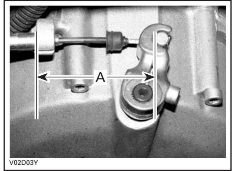
A. 68 à 75 mm (2-11/16 à 2-31/32 po)
