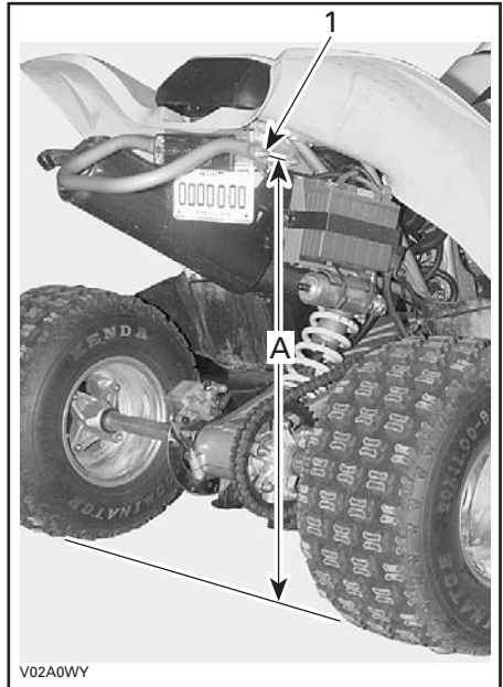
1. Écrou du pare-chocs arrière
