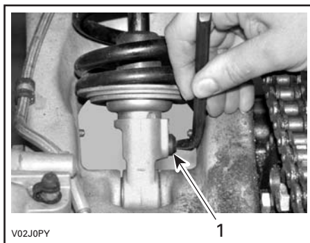
1. Ajusteur
