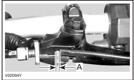
A. 3.5 ± 0.5 mm (9/64 ± 1/64 po)
