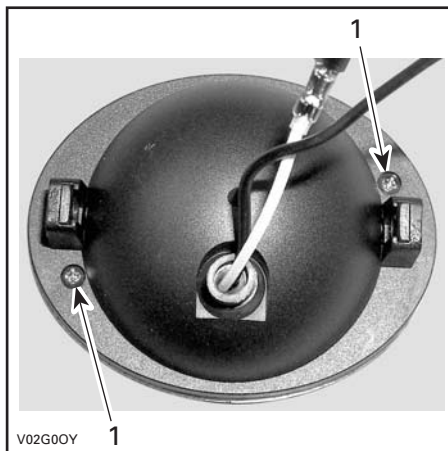
1. Retirer ces vis
