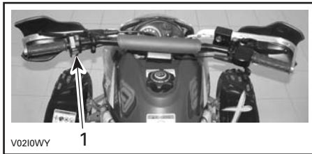
1. Interrupteur multifonctionnel
