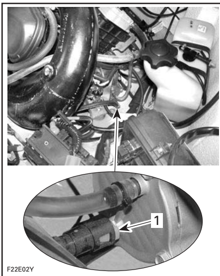
1. Appuyer sur les languettes et débrancher le boyau
