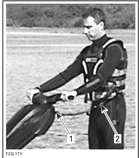
1. Capuchon sur la borne du cordon de sécurité 2. Cordon de sécurité fixé au VFI du conducteur
