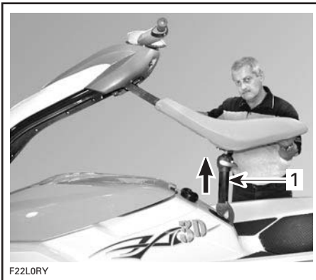
1. Montant du siège à la verticale
