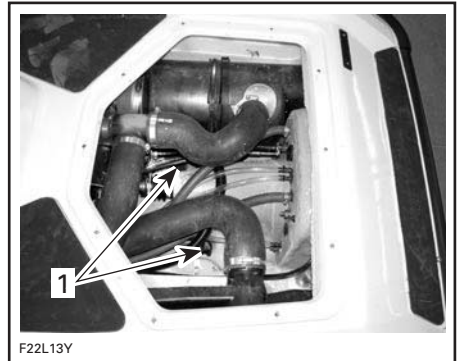
1. Siphons de cale automatiques
