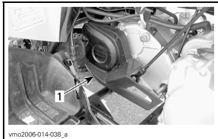
1. Drivkjedebeskyttelse
