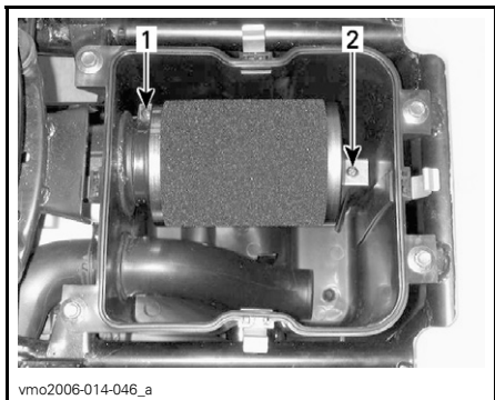
1. Klemme 2. Festeskruer
