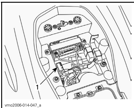
1. Sikringsholder
