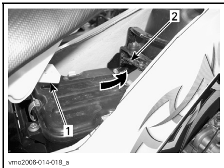
1. Tapp 2. Krok
