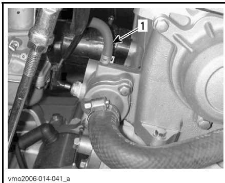
1. Forbløfingslange
