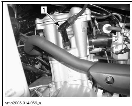
VENSTRE SIDE AV MOTOREN
