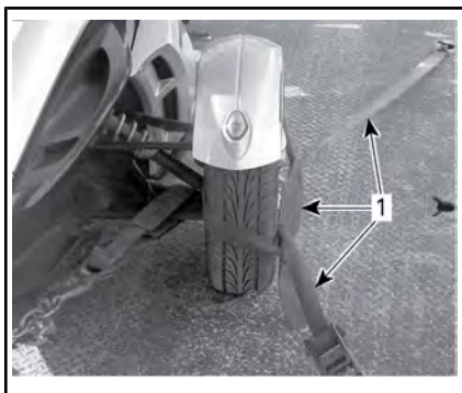
AGGANCIAMENTO RUOTE ANTERIORI — CONFIGURAZIONE TIPICA METODO 2
