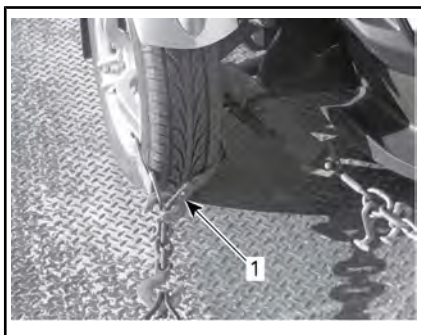
AGGANCIAMENTO RUOTE ANTERIORI — CONFIGURAZIONE TIPICA METODO 1
