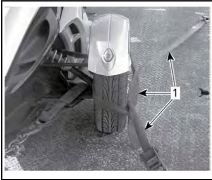
TÍPICO - SUJECIÓN DE LAS RUEDAS DELANTERAS
