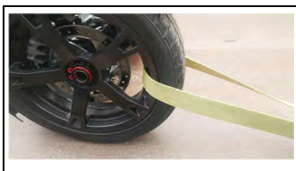
RUEDA DELANTERA
