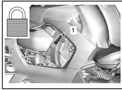
1. PARK-Hebel in der gesperrten Position (eingestellt)
