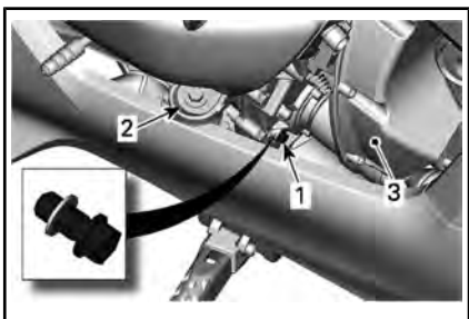
LAGE DER GETRIEBEÖLSTANDSKONTROLLSCHRAUBE
