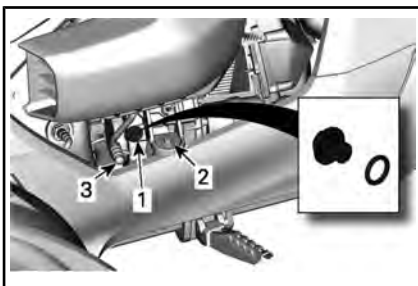
LAGE DER GETRIEBEÖLEINFÜLLSCHRAUBE
