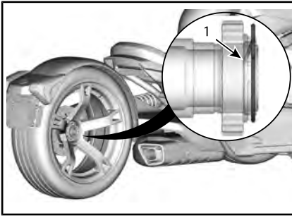
1. Umgebogenes Ende zeigt in die Antriebsachse
