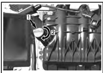
Schritt 1: Ölmesstab einstecken Schritt 2: Ziehen Sie den Ölmesstab fest.
