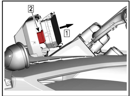
手順1：ゲージを取り外す 手順2：接続を切り離す
