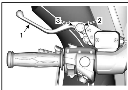
代表例 - クラッチレバーの調整
