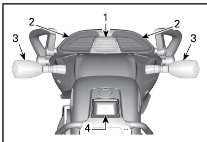
代表例-ライトの位置 — 車両後部 — すべてのモデル、ただし F3 リミテッドおよび F3-T、北米および日本向けモデルを除く
