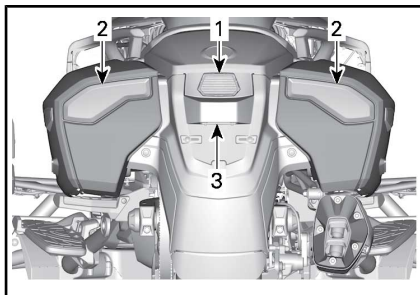
代表例-ライトの位置 — 車両後部 - F3-T モデル - すべての国向け
