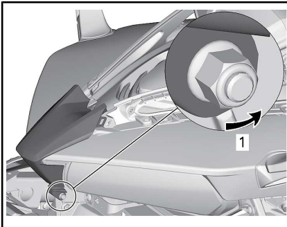
代表例 - コンソールノーズ(ピボット)
