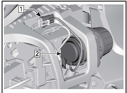
代表例 - ライトの位置 — 車両後部 - F3リミテッドモデル - すべての国向け
