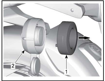
1. LED テールライトユニット 2. テールライトハウジング
