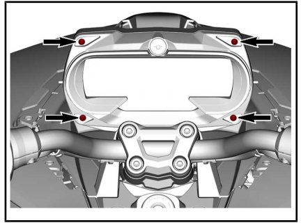
取り外すべき取り付けスクリュー
