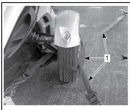
AGGANCIAMENTO TIPICO ALLE RUOTE ANTERIORI — METODO 2
