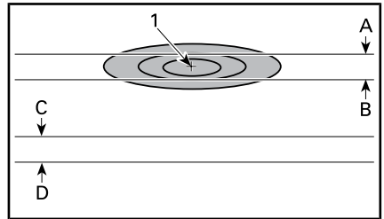
TYYPILLINEN – AJOVALON HEIJASTUS TESTIPINNALLA – KAUKOVALO (YKSI AJOVALO)
