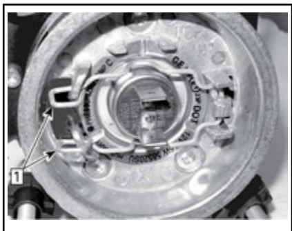
Vaihe 1: Vapauta jousipidikkeet
