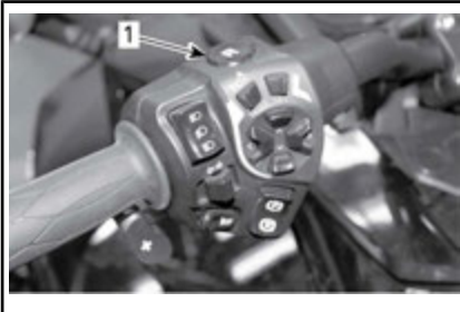
1. Umkehrmechanismus
