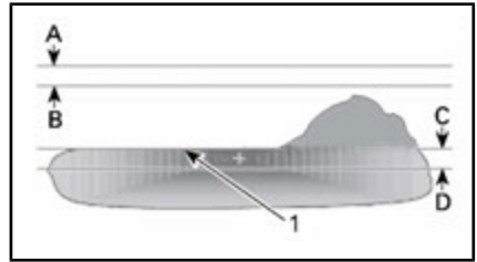
SCHEINWERFERREFLEKTION AUF TESTOBERFLÄCHE — ABBLENDLICHT (EINZELSCHEINWERFER)
