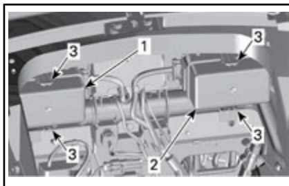
IM VORDEREN STAUFACH
