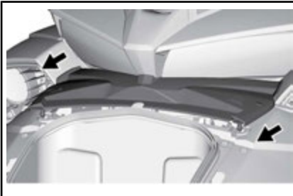
TYPISCH - WARTUNGSABDECKUNG ENTFERNEN
