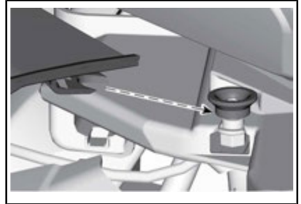
TYPISCH - HALTELASCHEN AN DER RICHTIGEN EINBAUSTELLE AUSRICHTEN
