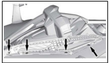
TYPISCH - ZU ENTFERNENDE BEFESTIGUNGSSCHRAUBEN
