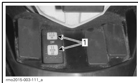
1. Interrupteur de poignées chauffantes du conducteur (en option)
