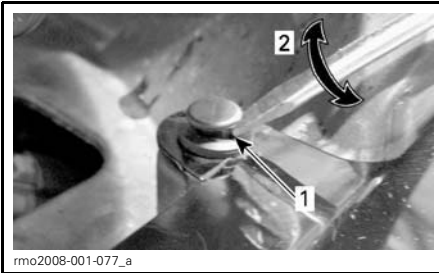
1. Tournevis à tête plate sous la tête du rivet 2. Tournez le tournevis de 1/4 de tour
