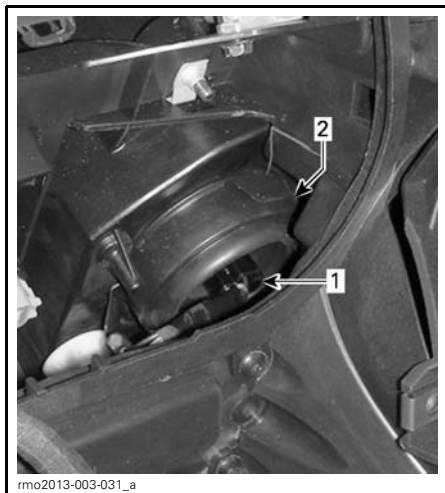
1. Connecteur électrique 2. Soufflet de caoutchouc
