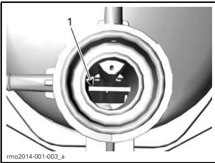
1. Ligne de référence de niveau de liquide de refroidissement (marque «HOT»)
