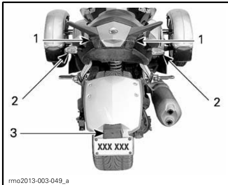
TYPIQUE - EMPLACEMENT DES FEUX – ARRIÈRE DU VÉHICULE
