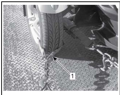
TYPISCH BEVESTIGING VAN DE VOORWIELEN — METHODE 1
