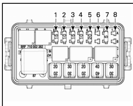
ZEKERINGEN - VERZEKERINGSDOOS RECHTS
