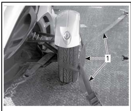
TYPISCH BEVESTIGING VAN DE VOORWIELEN — METHODE 2
