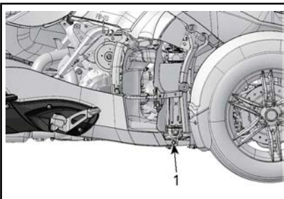
1. Voorste borgmoer
