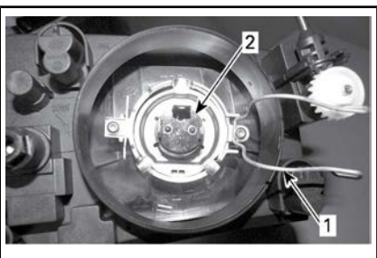
1. Lampveer 2. Lampbehuizing
