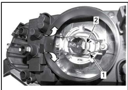
1. Lampveer 2. Lampbehuizing
