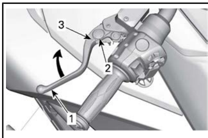
代表例 - クラッチレバーの調整
