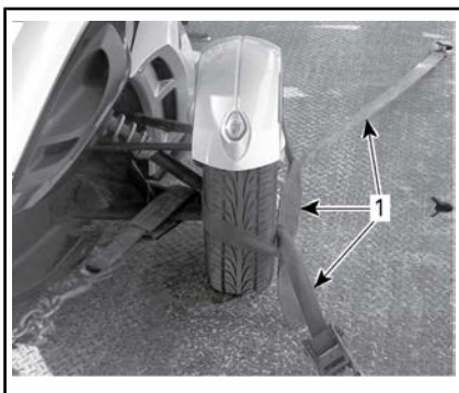
前輪の固定方法 — 代表例
