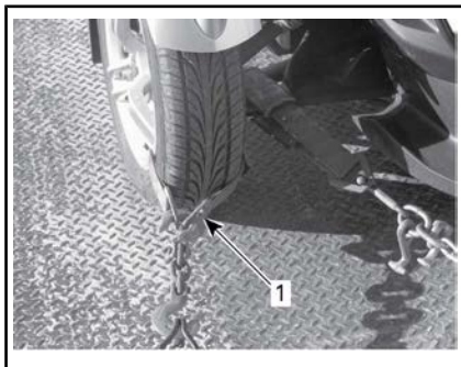
前輪の固定方法 — 代表例
