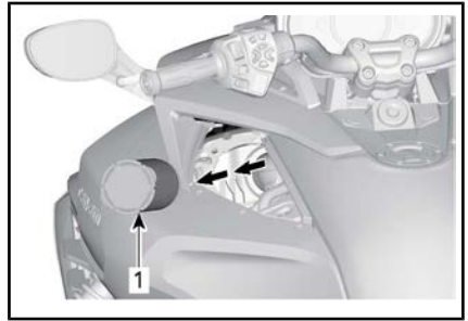
TYPEBILDE - DEMONTER LUFTFILTERET FRA LUFTINNTAKSDEMPEREN.
