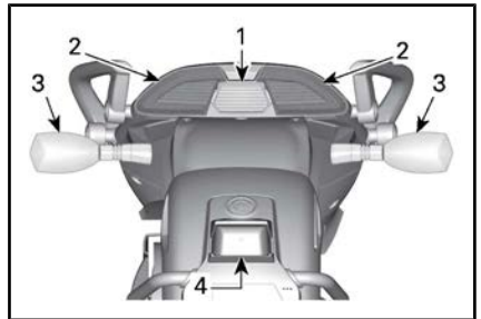
TYPEBILDE - PLASSERING AV LYS — BAK PÅ KJØRETØYET — ALLE MODELLER BORTSETT FRA NORDAMERIKANSKE OG JAPANSKE MODELLER SAMT LIMITED- OG T-MODELLER
