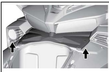
TYPEBILDE - LØFTING AV SERVICEDEKSEL
