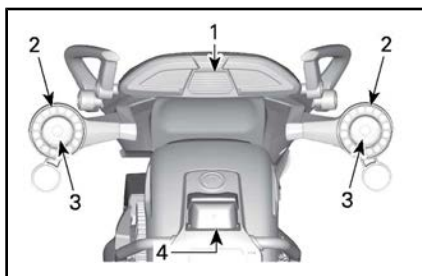
TYPEBILDE - PLASSERING AV LYS — BAK PÅ KJØRETØYET — JAPANSKE MODELLER AV F3 BASE OG F3-S
