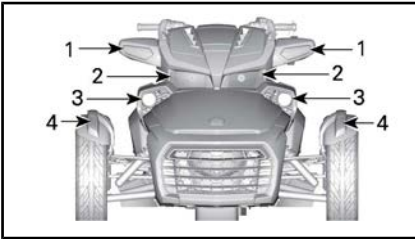
TYPEBILDE - PLASSERING AV LYS — FORAN PÅ KJØRETØYET — EUROPEISKE, AUSTRALSKE OG JAPANSKE MODELLER AV T OG LIMITED
