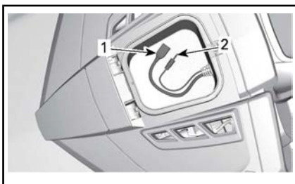
TYPEBILDE – DELER FJERNET FOR KLAR VISNING AV HANSKEROM
