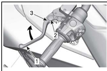
TYPEBILDE - JUSTERING AV CLUTCH-HÅNDTAK
