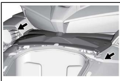
TYPEBILDE - AVTAKNING AV SERVICEDEKSEL
