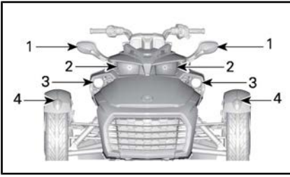
TYPEBILDE - PLASSERING AV LYS — FORAN PÅ KJØRETØYET — EUROPEISKE, AUSTRALSKE OG JAPANSKE MODELLER AV F3 BASE OG F3-S
