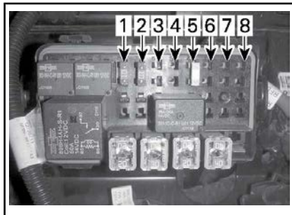
FUSIBLES: CAJA DE FUSIBLES DERECHA
