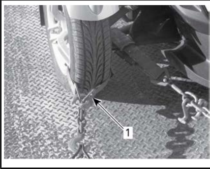
TÍPICO - SUJECIÓN DE LAS RUEDAS DELANTERAS
