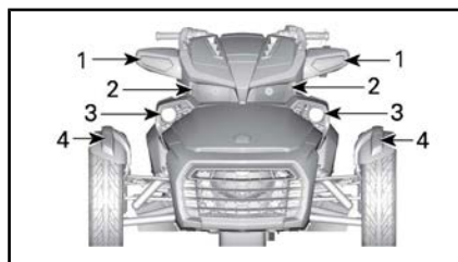
TÍPICO - UBICACIÓN DE LAS LUCES — PARTE DELANTERA DEL VEHÍCULO — MODELOS T Y LIMITADOS EUROPEOS, AUSTRALIANOS Y JAPONESES
