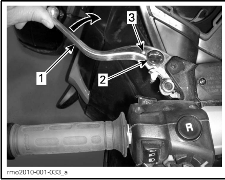
RÉGLAGE DU LEVIER D'EMBRAYAGE
