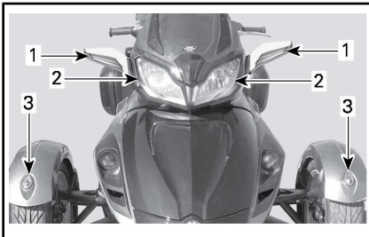
TÍPICA - LOCALIZAÇÃO DAS LUZE — FRENTE DO VEÍCULO
