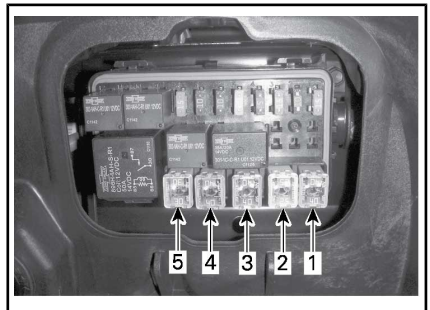
FUSÍVEIS JCASE - CAIXA DE FUSÍVEIS ESQUERDA
