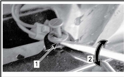
1. Chave de fenda sob o rebite 2. Gire a chave de fenda em 1/4 de volta 3. Desligue os conectores do corpo da seta direita. 4. Retire o parafuso Torx atrás da lente, como indicado abaixo.
