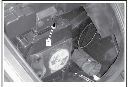
TAMPA DO TANQUE NO LADO ESQUERDO ABAIXO DO ASSENTO
