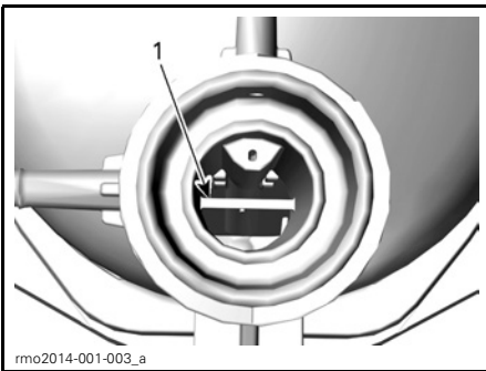
1. Ligne de référence du niveau du liquide de refroidissement
