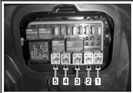
FUSIBLES JCASE - CAJA DE FUSIBLES IZQUIERDA
