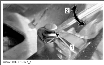
1. Destornillador de cabeza plana debajo de cabeza de remache 2. Haga girar el destornillador 1/4 de vuelta
