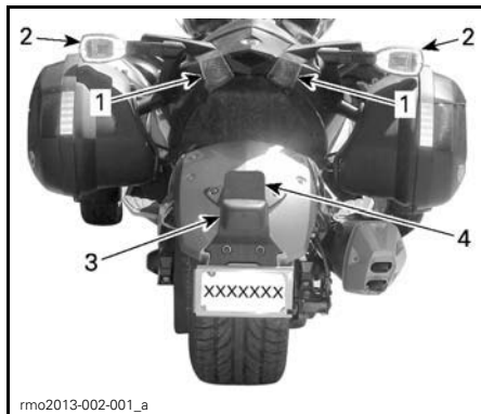
TYPIQUE - EMBLACEMENT DES FEUX — ARRIÈRE DU VÉHICULE
