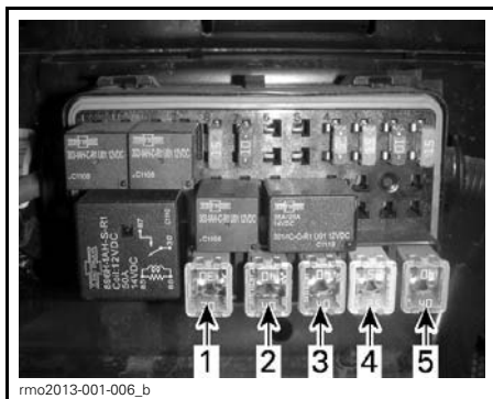
FUSIBLES JCASE - BOÎTE À FUSIBLES GAUCHE
