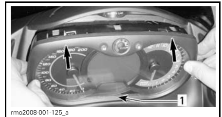
INSTALLATION DU TABLEAU DE BORD 1. Insérez le rebord inférieur d'abord puis appuyez sur le rebord supérieur
