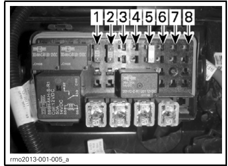
FUSIBLES - BOÎTE À FUSIBLES DROITE
