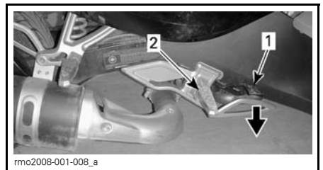
1. Jarrupoljin 2. Astinlauta (jalkatuki)
