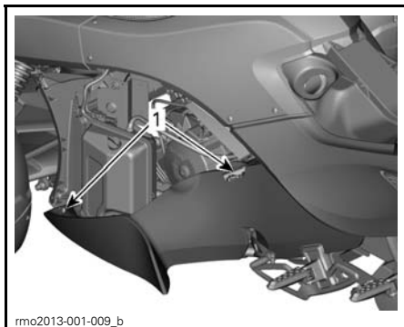
1. Takaosan alasisivupaneelin Torx-ruuvit
