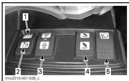
1. Interruptor del compartimento de almacenamiento delantero
