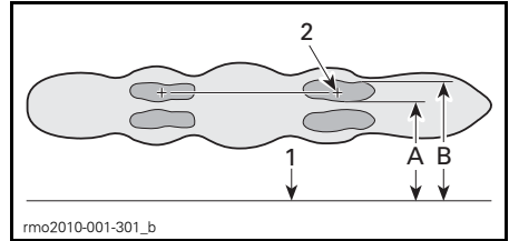
TYPISCHE LICHTBUNDEL VAN DE KOPLAMPEN OP HET TESTOPPERVLAK
