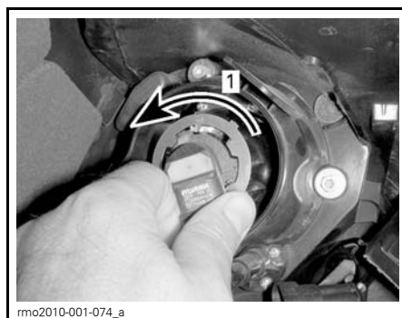
1. Draai linksom
