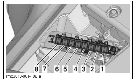
ZEKERINGEN ONDER HET ZADEL
