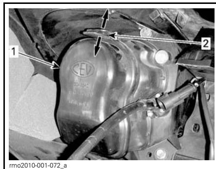
1. Deksel koplamp 2. Trek de lipjes uiteen
