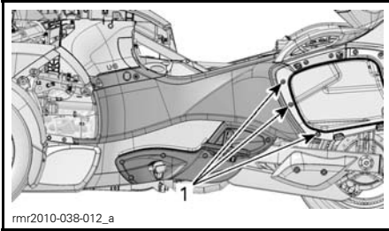
1. Achterste borgschroeven
