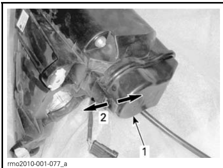
1. Deksel koplamp 2. Trek de lipjes uiteen
