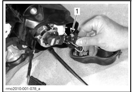
1. Koppel de connector los
