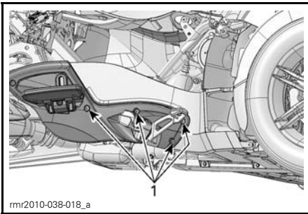
1. Kiinnitysruuvit
