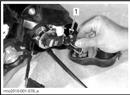
1. Irrota liitin
