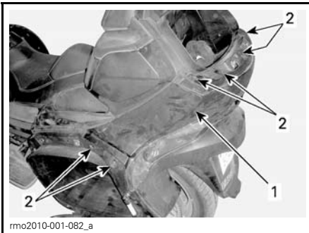
1. Takapaneeli 2. Kiinnitysruuvit
