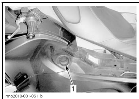
1. Polttoainesäiliön korkki
