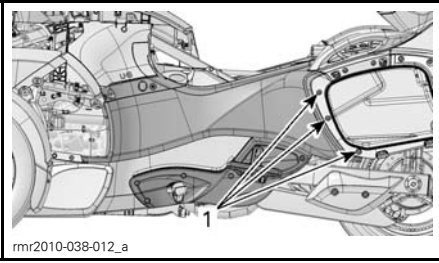
1. Takakiinnitysruuvit
