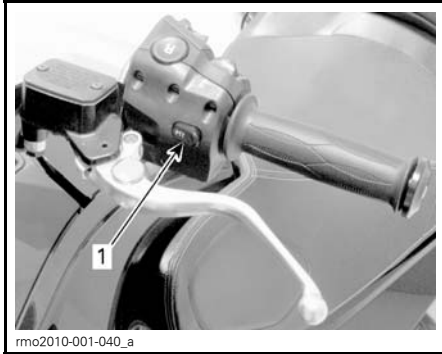
1. PTT-Taster
