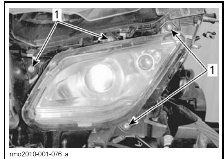
1. Befestigungsschrauben
