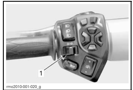
1. Blinkerschalter
