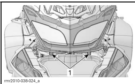
1. Untere Befestigungsschraube
