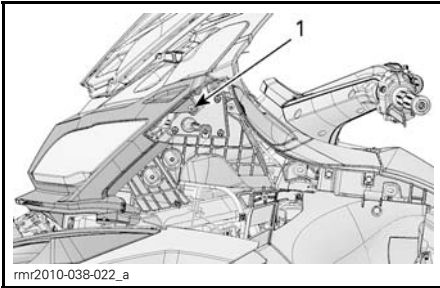
1. Obere Befestigungsschraube
