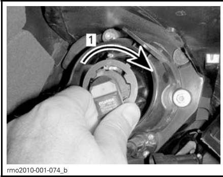
1. Draai rechtsom
