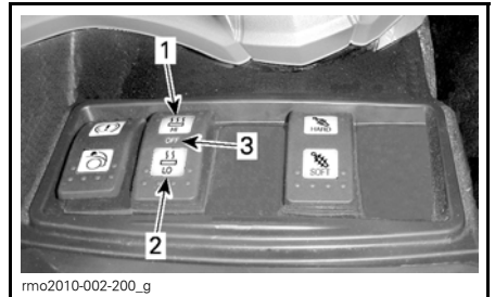
1. HI Maximumintensiteit 2. LO Minimumintensiteit 3. OFF (Uit) (middelste stand)
