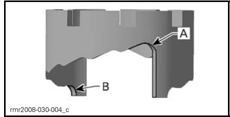
A. Zachte afstelling (stand 1) B. Harde afstelling (stand 5)
