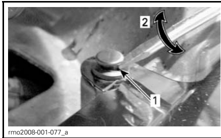
1. 2 rivets de plastique sous le siège
