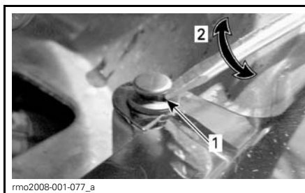
1. Tournevis plat sous la tête du rivet 2. Tournez le tournevis de 1/4 de tour
