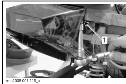
1. Retirez la vis Torx derrière la lentille
