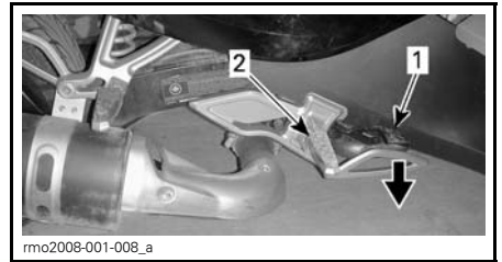
1. Jarrupoljin 2. Jalkatappi
