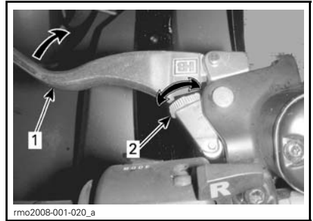
KYTKINVIVUN SÄÄTÖ
