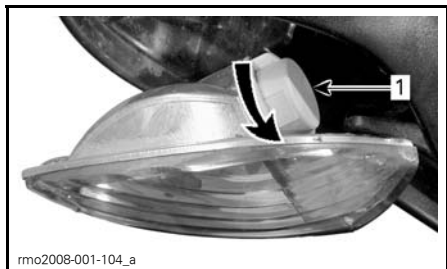
1. Etusuuntavilkun liitin
