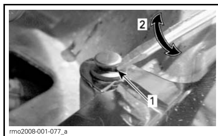
1. 2 Kunststoffniete unter dem Sitz
