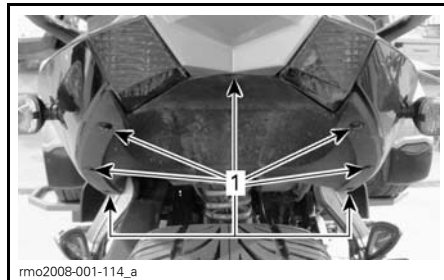
VERKLEIDUNG UNTER DEM BEIFAHRERSITZ 1. Anordnung der 7 Torx-Schrauben
