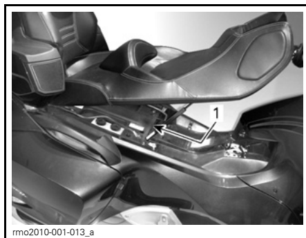
1. Caixa de fusíveis localizada sob o assento
