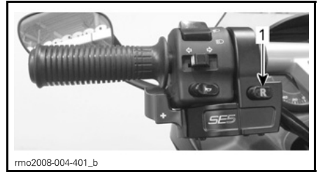
1. Botón de marcha atrás
