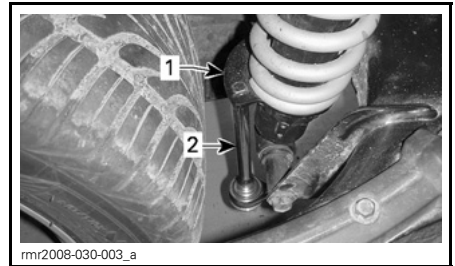
1. Ajustador de leva 2. Trinquete con extensión
